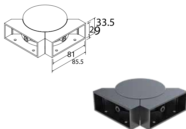
CODICE: 4375 CONNETTORE AD ANGOLO PER CORRIMANO CLS- 201/FSN-221
