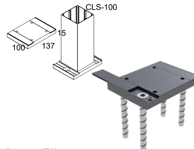
CODICE: 4741 SUPPORTO PER COLONNA CLS-100 CON 4 VITI
