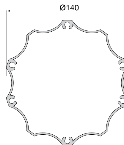
CODICE: 67 PESO: 3153 gr/m COLONNA 140X140
