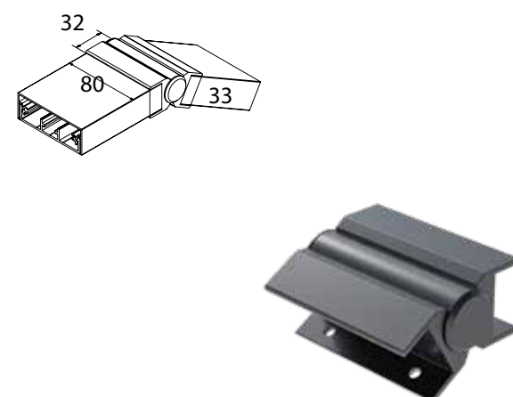
CODICE: 4379 CONNETTORE ORIENTABILE PER CORRIMANO CLS-202
