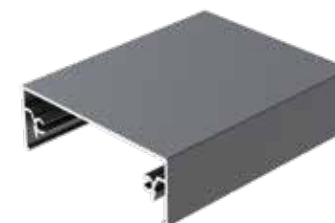
CODICE: FSN-221 PESO: 754 gr/m COVER PER CORRIMANO 80x28
