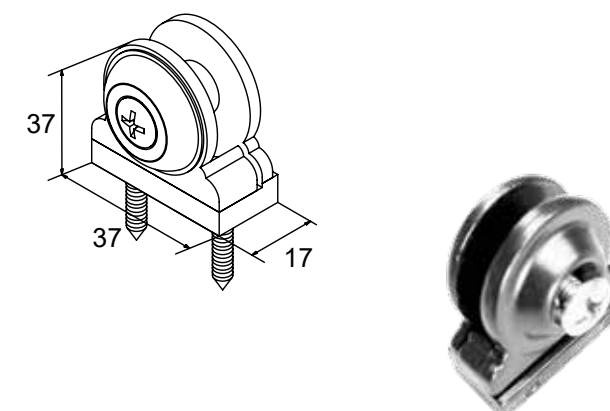
CODICE: 24 ATTACCO PER GUIDA AL-FLEX
