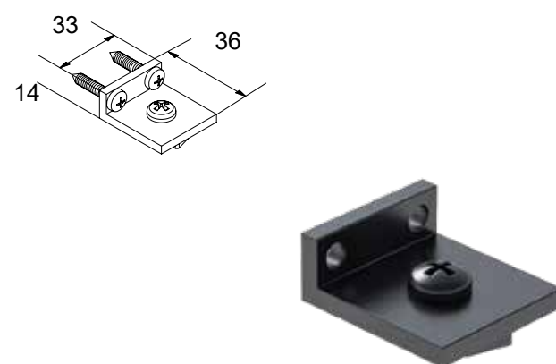
CODICE: 4272 CONNETTORE PER GUIDA CLS-306
