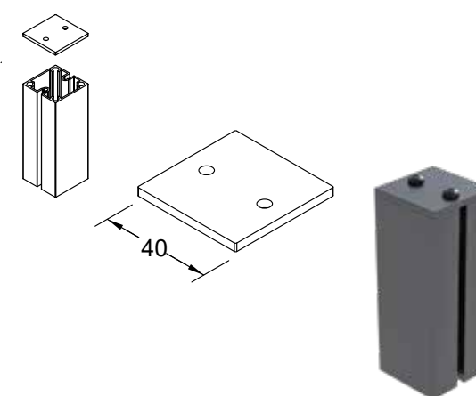
CODICE: 4489 TAPPO PIATTO PER COLONNA CLS-103 (40x40)
