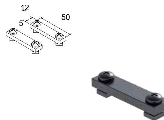
CODICE: 4278 CONNETTORE PER GUIDA CLS-303
