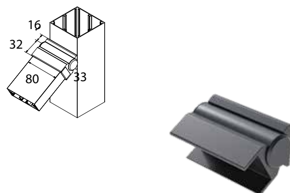
CODICE: 4378 CONNETTORE PER CORRIMANO FSN-221 E COLONNA CLS- 100
