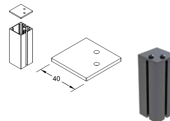
CODICE: 4490 TAPPO PIATTO PER COLONNA CLS-104 (40x40)
