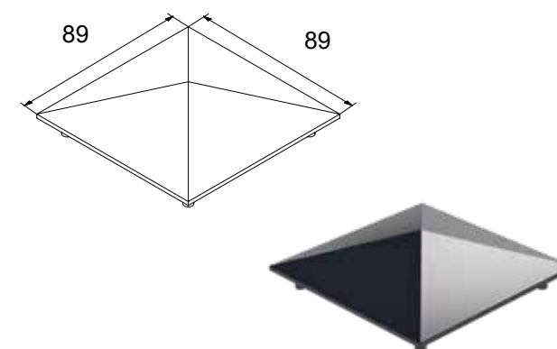
CODICE: 4485 TAPPO DECORATO PER COLONNA CLS-100
