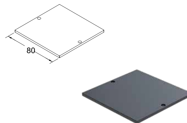
CODICE: 4486 TAPPO PIATTO PER COLONNA CLS-100 (80x80)
