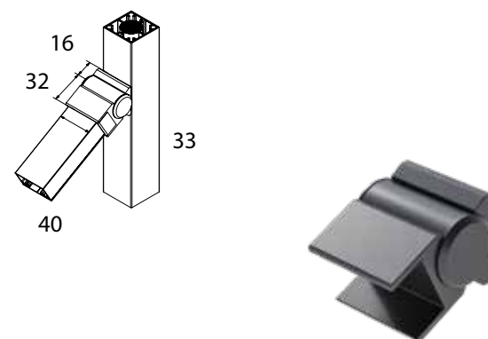
CODICE: 4377 CONNETTORE PER GUIDA CLS-3K2 CON COLONNA CLS-102
