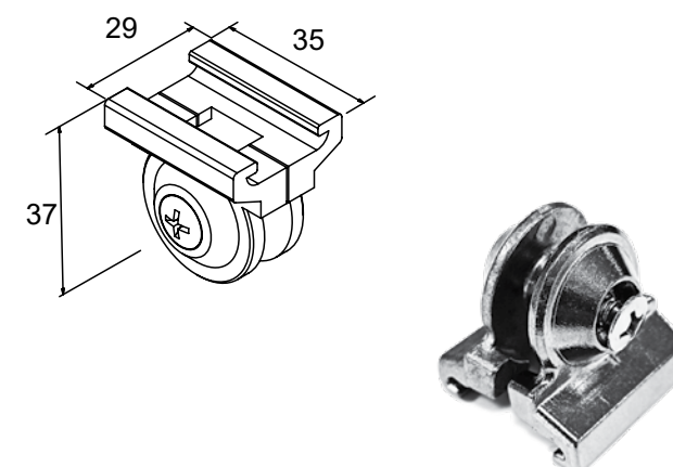
CODICE: 22 ATTACCO PER GUIDA AL-FLEX
