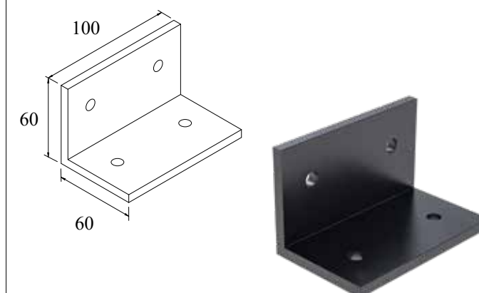
CODICE: 4282 SUPPORTO A MURO PER COLONNA CLS-102
