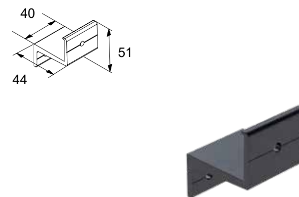
CODICE: 4274 SUPPORTO ESTERNO PSATHA
