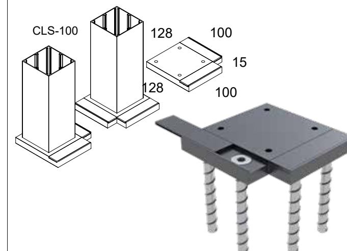
CODICE: 4742 SUPPORTO PER COLONNA CLS-100 CON 4 VITI
