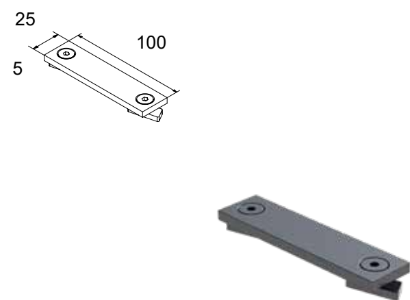
CODICE: 4261 CONNETTORE PER CORRIMANO
