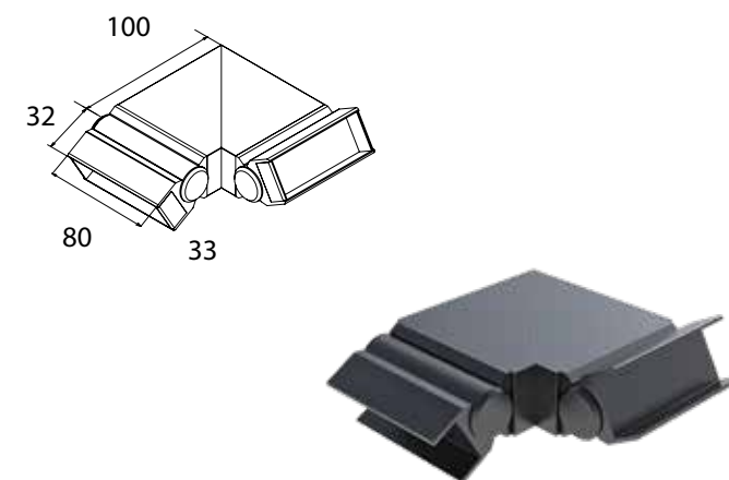
CODICE: 4384 CONNETTORE AD ANGOLO 90° PER CORRIMANO CLS-202 (SCALE)
