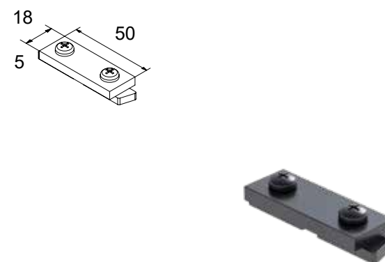
CODICE: 4275 CONNETTORE PER GUIDA CLS-302
