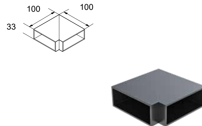
CODICE: 4273 CONNETTORE AD ANGOLO PER CLS-201/FSN-221
