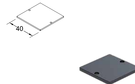
CODICE: 4487 TAPPO PIATTO PER COLONNA CLS-102 (40x40)
