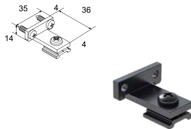
CODICE: 4270 CONNETTORE PER CLS-201/301/302/305
