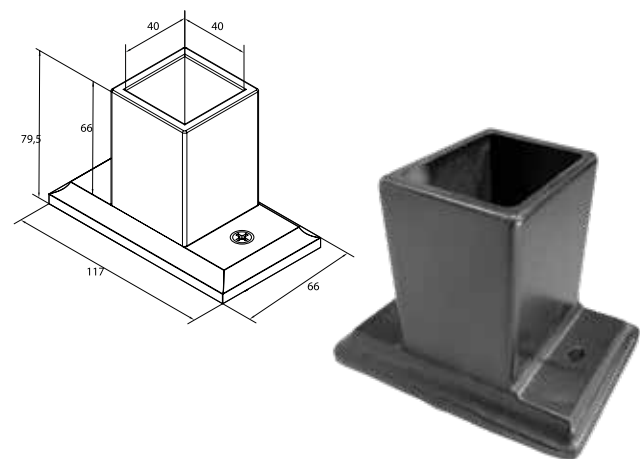
CODICE: 4113 SUPPORTO PER COLONNA 40x40
