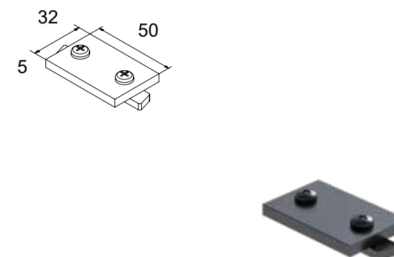
CODICE: 4276 CONNETTORE PER GUIDA CLS-306
