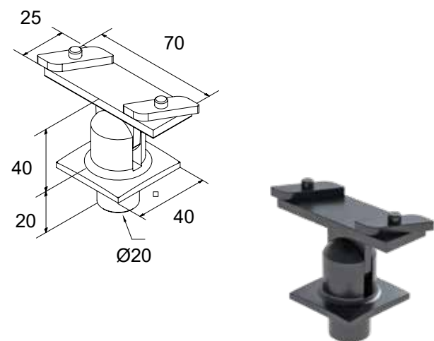
CODICE: 4345 CONNETTORE PER COLONNA CLS-102 E CORRIMANO F50-201
