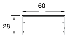
CODICE: CLS-307 PESO: 262 gr/m GUIDA PER RINGHERE AL-FLEX
