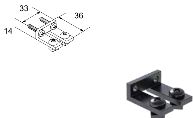
CODICE: 4271 CONNETTORE PER GUIDA CLS-303
