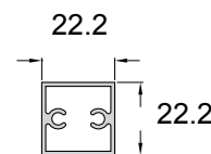
CODICE: FSN-221 PESO: 754 gr/m COVER PER CORRIMANO 80x28
